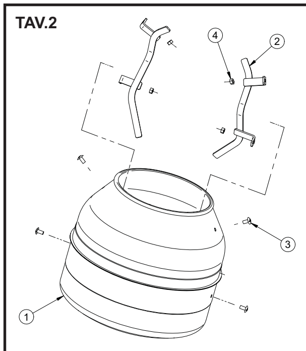
TAV.2 VASCA IN ACCIAIO - CUVE EN ACIER - STEEL DRUM - MISCHTROMMEL AUS STAHL - CUBA DE ACERO
